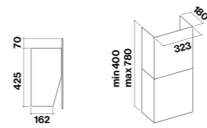
Zijaanzicht
