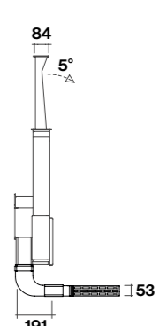
Plint rooster, voor gebruik met filter KACL.951 h60 (optioneel)
