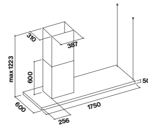
Linker versie
