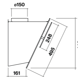
Zijaanzicht
