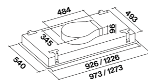
Externe doorvoer motor KACL.798#41F
