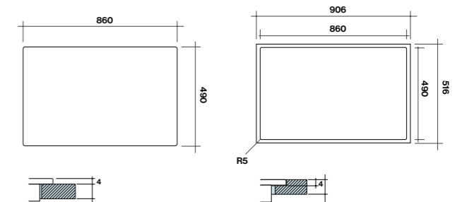
Opbouw afmetingen
