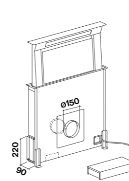
Installatie voorbeelden.
