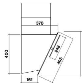
Zijaanzicht
