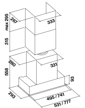
Uitsparing: 50 cm: 506 mm x 262 mm 70 cm: 751 mm x 262 mm
