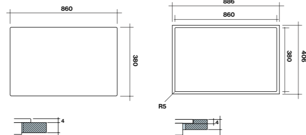
Opbouw afmetingen
