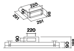
Aansluitstuk (KACL.789)
