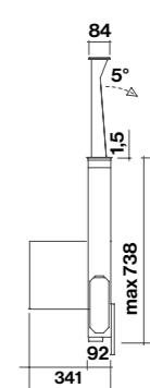
Zijaanzicht, motor aan achterkant
