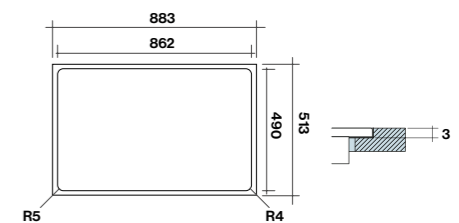
Vlak inbouw Gatmaat
