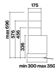
Zijaanzicht met optionele schacht
