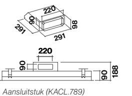
Aansluitstuk (KACL.789)
