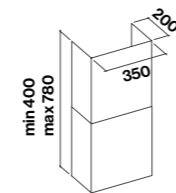
Schacht optioneel
