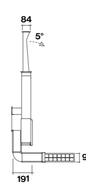
Zijaanzicht, Slim motor achter
