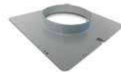
Flens voor krachtigere motoren (1500 - 1300 m 3 /h) KACL.396 ø200
