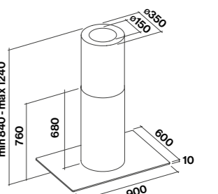
Eiland versie met glas (optioneel)
