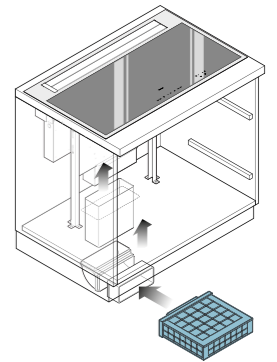
Koolstof Zeoliet filter versie Plint (KACL.930)
