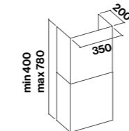
Schacht optioneel
