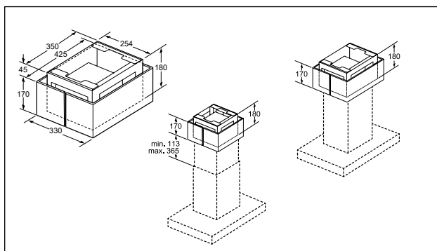
Schéma Set CleanAir Plus pour hottes îlot
