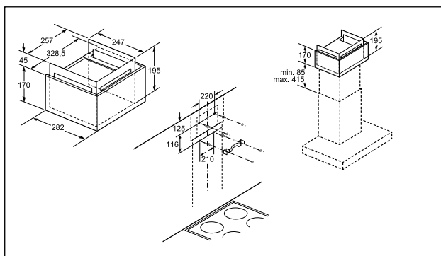
Schéma Set CleanAir Plus pour hottes murales
