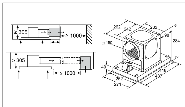
Schéma Set CleanAir Plus pour extracteur d'air
