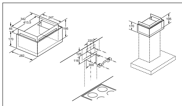
Schéma Set CleanAir Plus pour hottes murales
